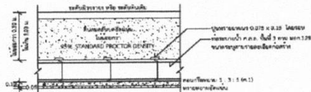
รูปตัด ก-ก
