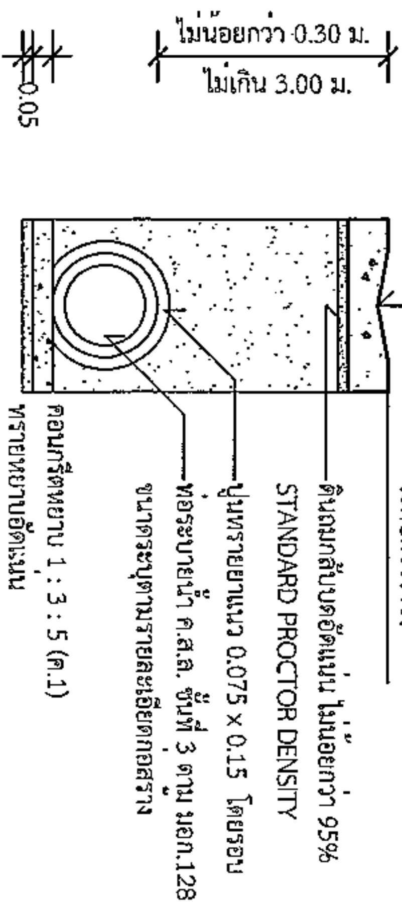
กรณีวางท่อกลมมีรางขึ้น
