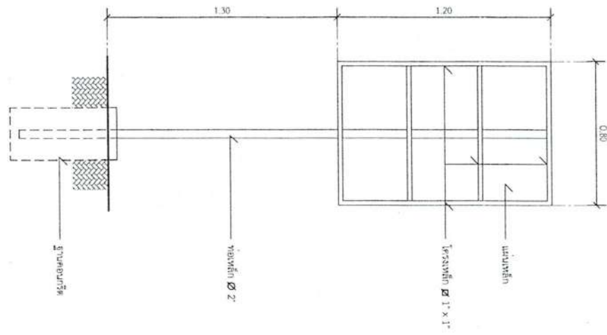
รูปด้านบน 1 : 20
